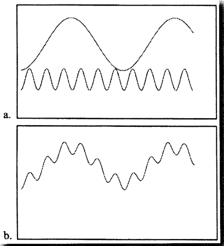
Kuva 3. Esimerkki Fourier- eli taajuusanalyysistä, jossa aikasarjat voidaan esittää harmonisten komponenttien eli eri vaihteisten ja taajuisten siniaaltojen summana. Kuvassa 3a on kaksi siniaaltoa, joista ylempi on taajuudeltaan matalampi ja alempi taajuudeltaan tiheämpi. Jos nämä kaksi sinikäyrää lasketaan yhteen, saadaan kuvan 3b kaltainen kuvio, jossa on nähtävissä kummankin sinikäyrän osuus.
