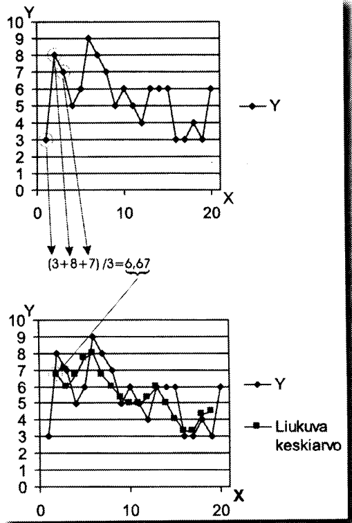
Kuva 1. Esimerkki kolmen pisteen liukuvan keskiarvon laskemisesta
